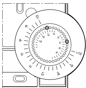
Afbeelding 6: Instelbereik begrenzen
